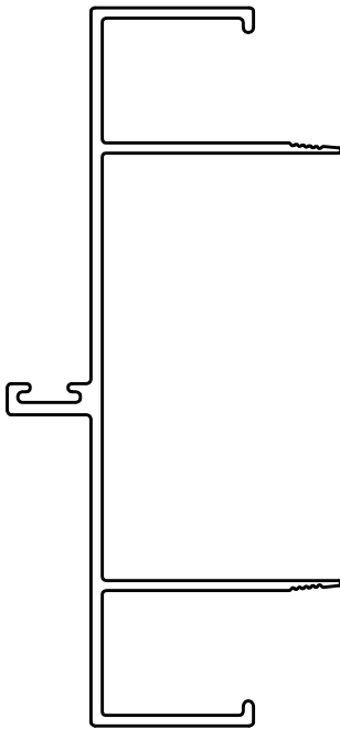
39383 DOOR FRAME 1
