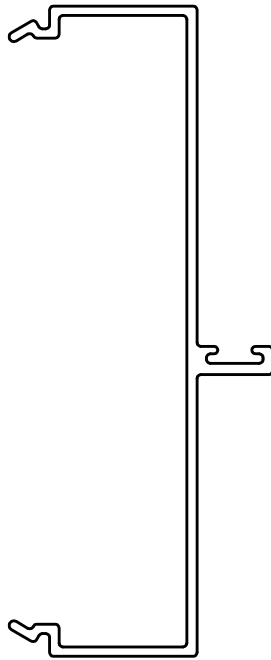
39381 DOOR FRAME 2
