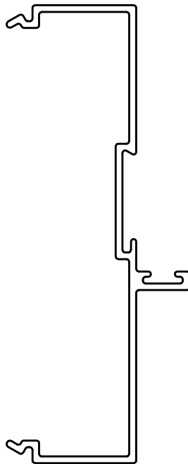
39380 GLAZING 2
