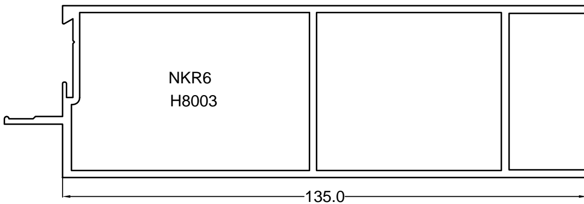
DOOR SECTIONS
